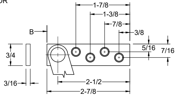
JAMB BRACKET
