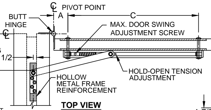
OFFSET PIVOT
