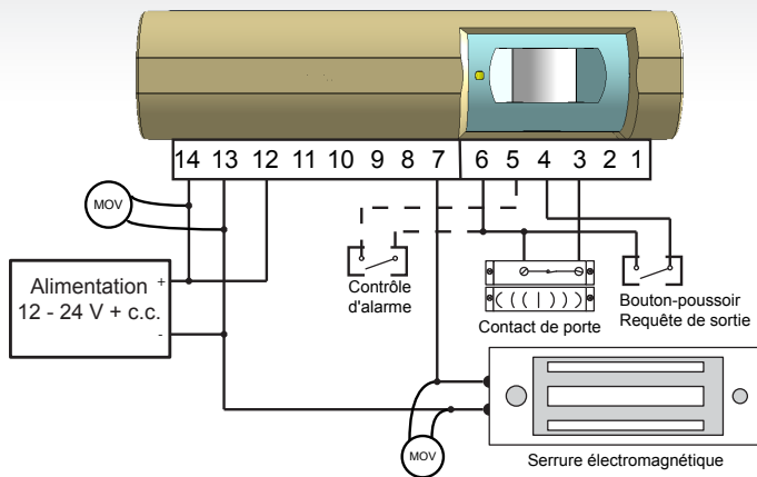
SCHÉMA DE CÂBLAGE DES MODES 1 ET 2
