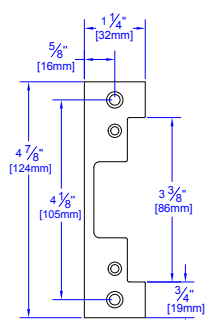
ESF1 - ANSI SQUARE
