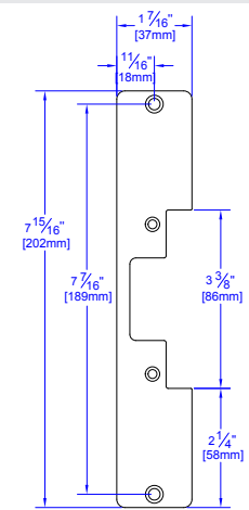
ESF4 - WOOD DOOR
