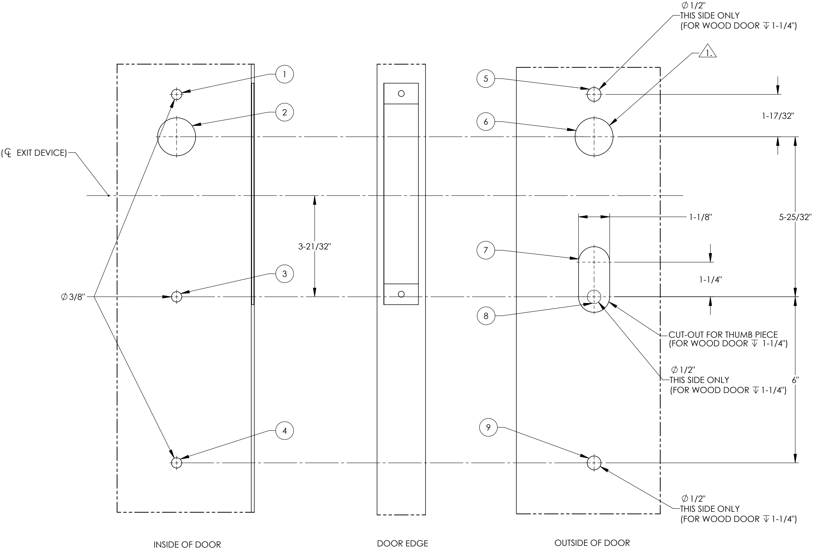
R.H.R.B. DOOR SHOWN
