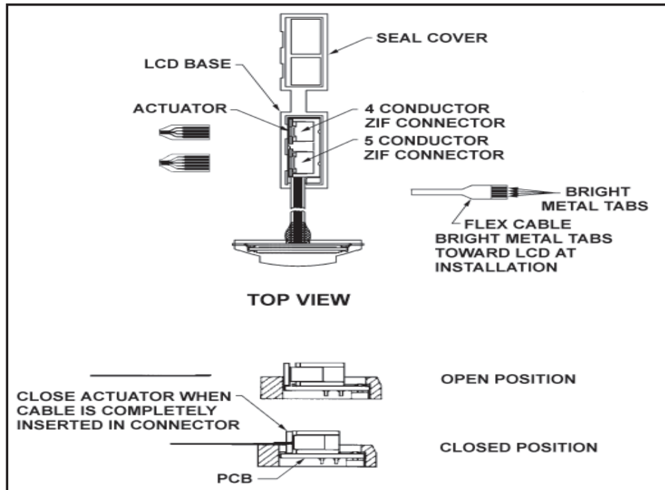
Figure 14 - LCD and ZIF connectors
