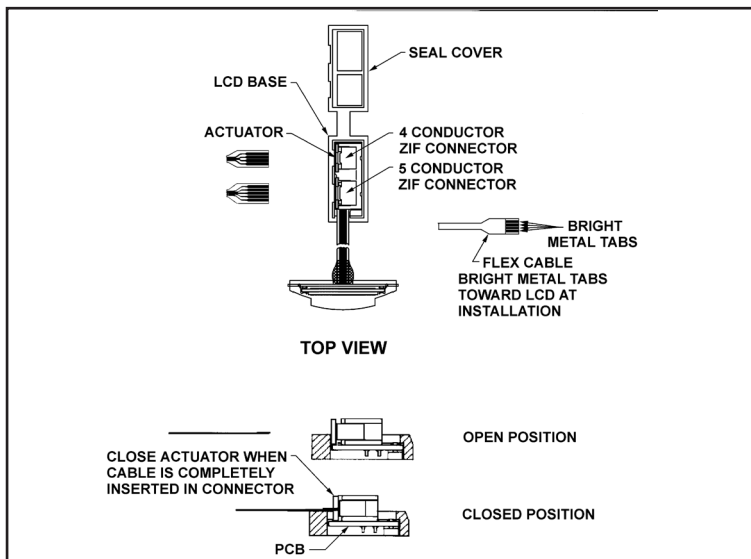
Figure 13 - LCD and ZIF Connectors
