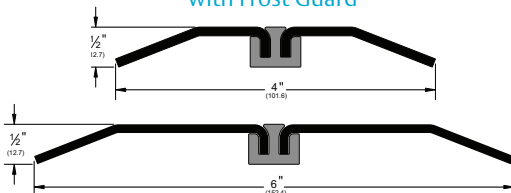
Door Bottom Sweep 315SSR
