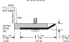
Perimeter Gasketing 305SSS
