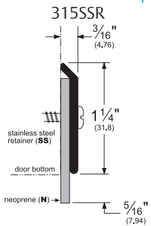
Door Bottom Sweep 315SSR
