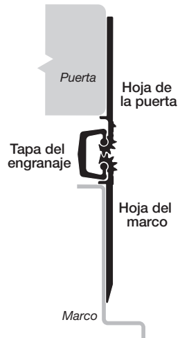
Fig. 3 Puerta abierta a 180°
