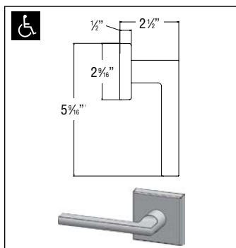
ORLANDO (ORL) (SPECIFY HANDING)
