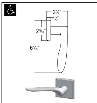
MEMPHIS (MEM) (SPECIFY HANDING)
